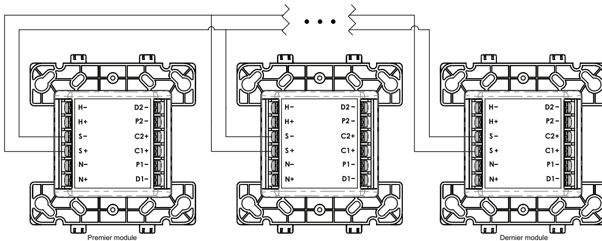
INTERCONNEXION DES MODULES DE SYNCHRONISATION (20 MODULES MAXIMUM) : Pour obtenir plus de précisions, consulter le manuel d'installation LT-6151
