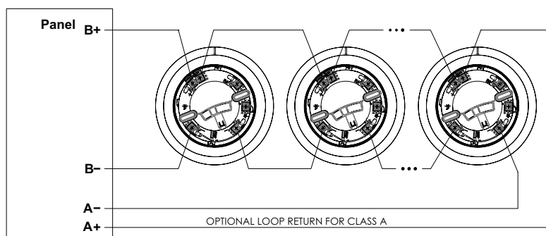
LOOP WIRING
