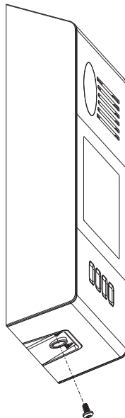
Figure 6. Fixer le TX3 Nano sur la plaque de montage
