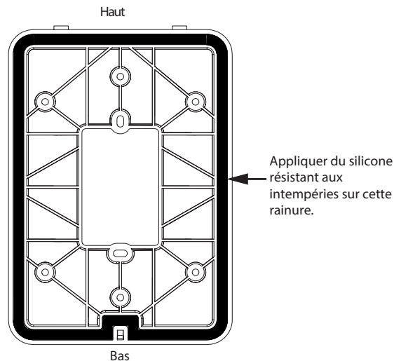
Figure 1. Plaque de montage par l'arrière : appliquer du silicone dans la rainure
