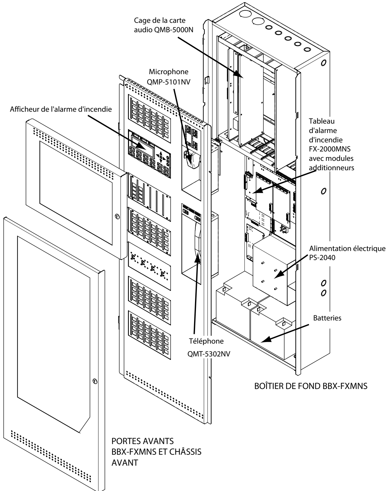
Figure 2: Vue élargie du boîtier BBX-FXMNS
