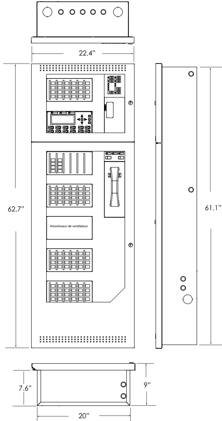
Figure 1: Boîtier BBX-FXMNS avec dimensions
