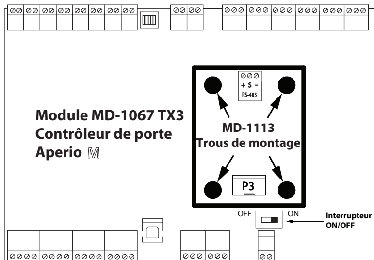
Figure 1. Emplacement des trous de montage du MD-1113 et du P3 (connecteur de modem).
