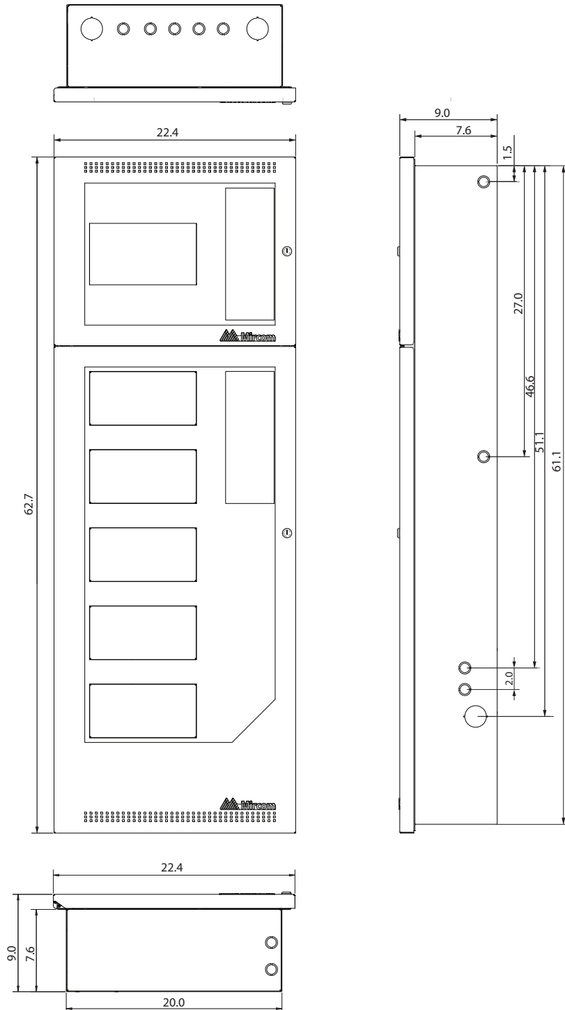
Figure 1: Boîtier BBX-FXMNSRG avec dimensions
