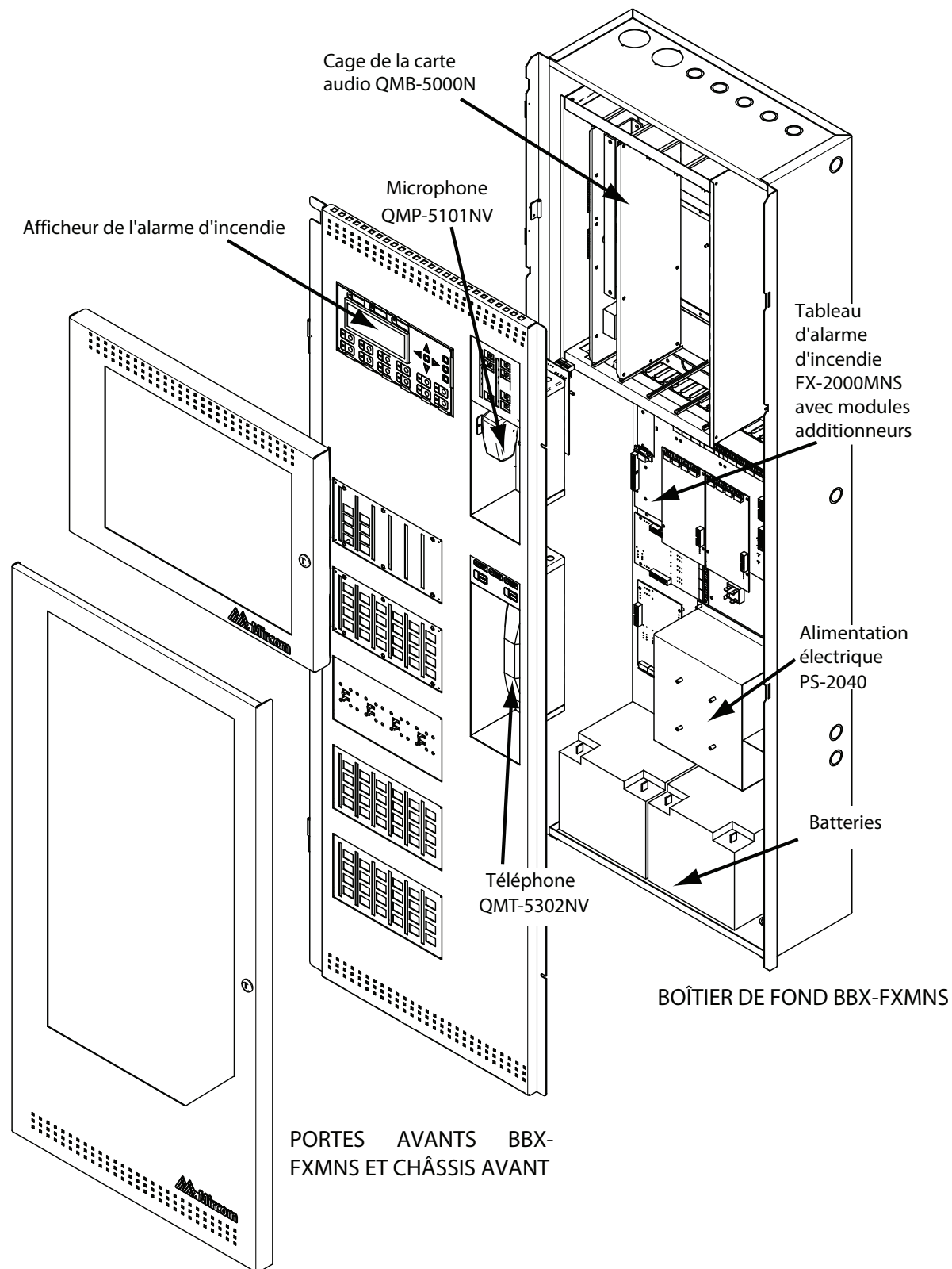
Figure 2: Vue élargie du boîtier BBX-FXMNSRG
